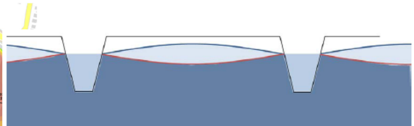
Figuur 3-11: Conceptuele weergave van een bolle (blauwe lijn) en holle grondwaterstand (rode lijn).
