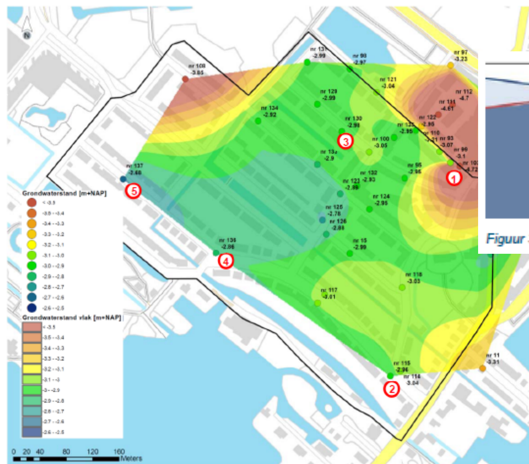
Figuur 3-4: Gemiddelde, fretische grondwaterstand periode 2012-2015 (Bron: grondwatermeetnet gemeente Rotterdam, 2015)
